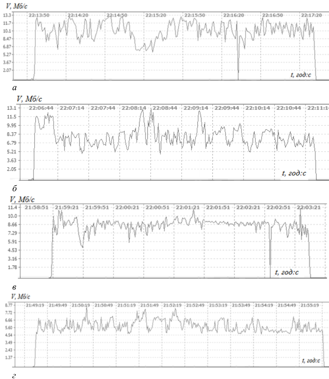
Рис. 2. Часові залежності ефективної швидкості передачі для каналу шириною 20 МГц при: прямій видимості (а); наявності перешкоди П1 (б); наявності перешкоди П1 та П2 (в); наявності перешкоди П2 та П2 (г)
