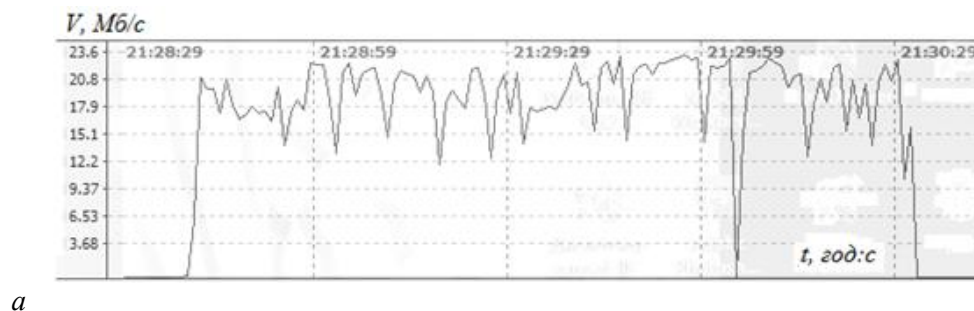
Рис. 2. Часові залежності ефективної швидкості передачі для каналу шириною 20 МГц при: прямій видимості (а); наявності перешкоди П1 (б); наявності перешкоди П1 та П2 (в); наявності перешкоди П2 та П2 (г)
