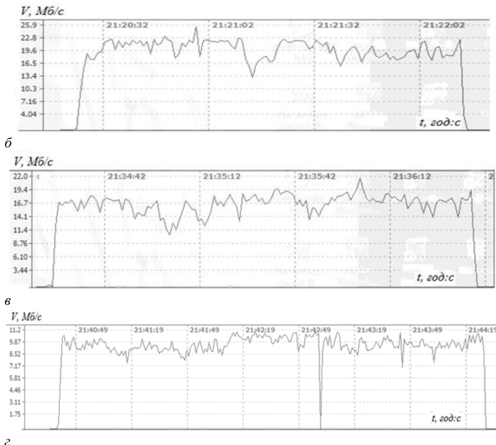
Рис. 3. Часові залежності ефективної швидкості передачі для каналу шириною 40 МГц при: прямій видимості (а); наявності перешкоди П1 (б); наявності перешкоди П1 та П2 (в); наявності перешкоди П2 та П2 (г)
